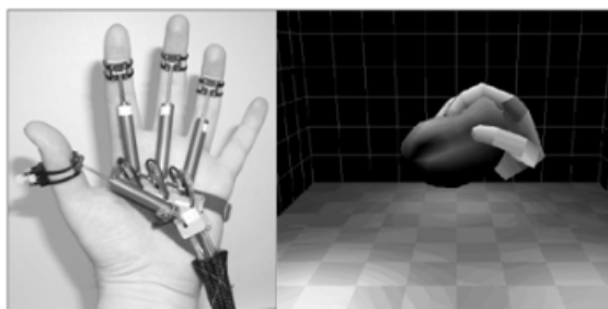
Figura 1 – Luva com sistema unificado de captura de movimento e emissão de força com exemplo de aplicação
