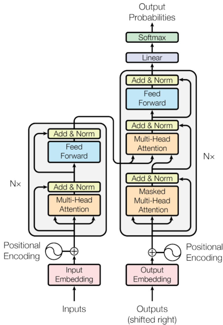
Hình 1: Kiến trúc của mô hình Transformer [1]
